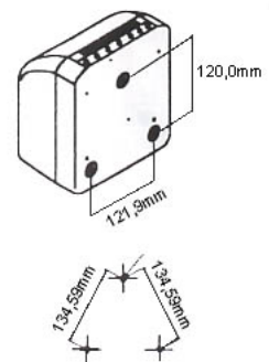
Position der einzelnen Aufhängungen
